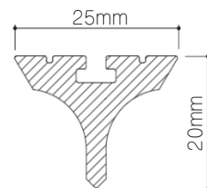
断面形状
