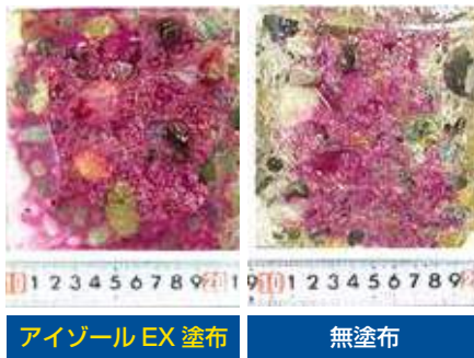
中性化促進試験(26週)の状況
