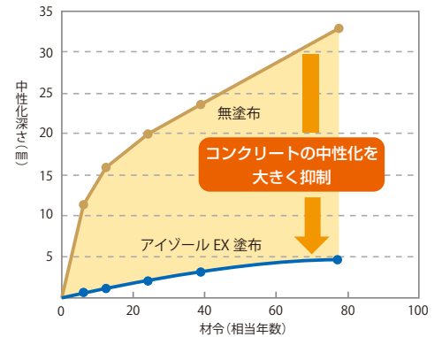
■ 中性化促進試験の一例(コンクリート強度: 24N/㎠)
