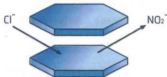
塩化物イオン吸着剤の構造模式図
